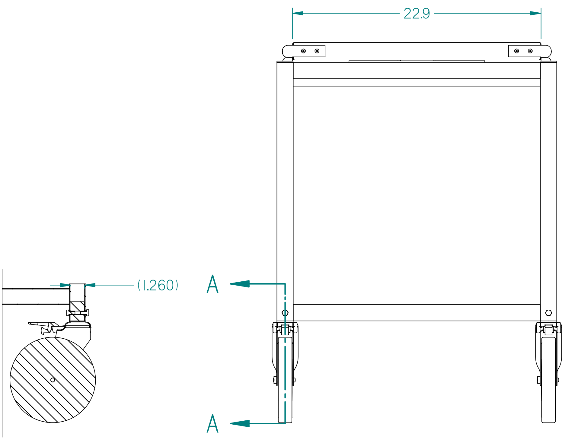
SECTION A-A
